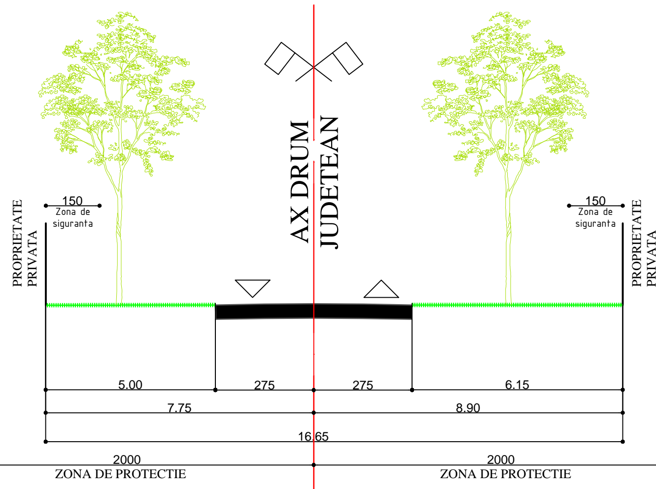
PROFIL DRUM JUDETEAN EXISTENT INTRAVILANUL LOCALITATII DJ 221 (Str. Saratei)
