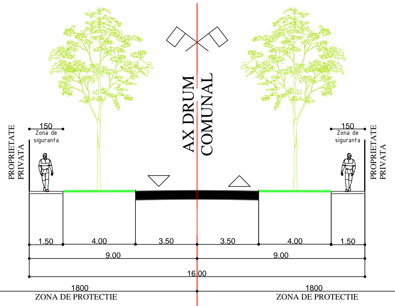
PROFIL DRUM COMUNAL EXISTENT IN IANCA DC35 (Str. Garii)
